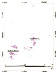
Şekil 27. Çalışılan alanda İkonos uydu verisinde K Means Sınıflama ile elde edilen görüntü.
