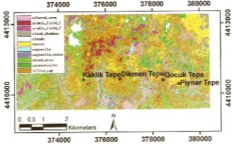
Şekil 29. İkonos genel görüntüsünden üretilen Maximum Likelihood sınıflandırma.
