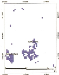
Şekil 3. Çalışılan alanda Landsat uydu verisinde FC Means Sınıflaması ile elde edilen görüntü.
