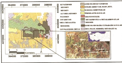
Şekil 1. Bölgenin yer bulduru ve 1/500.000 ölçekli basitleştirilmiş jeolojî haritası ve Landsat 531 kompozitindeki görünümü (MTA, 2001).
