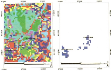
Şekil 7. Çubuklan alanda Landsat uydu verisinde K Means Sınıflaması ile elde edilen görüntü.
