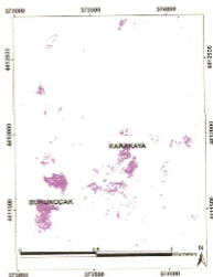
Şekil 25. Çalışılan alanda İkonos uydu verisinde FC Means Sınıflama ile elde edilen görüntü.
