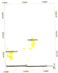
Şekil 14. Çalışılan alanda Aster uydü verisinde FC Means Sınıflaması ile elde edilen görüntü.
