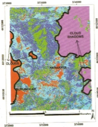
Şekil 23. Çalçalan alanında İkonos uydurisinde Adaptive Sınıflaması ile elde edilen görüntü.
