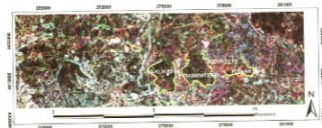
Şekil 33. Landsat RGB 531 görüntüsü kullanılarak elde edilen Edge Detection-kenar belirleme filtreleme görüntüsü. Sarı çizgi ile sınırlanmış alanlar silika'ca zengin silika kapakları, kırmızı çizgi ile çevrelenmiş alanlar manyezitce zengin alanları göstermektedir.
