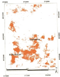
Şekil 21. Çalçalan alanında İkonos uydurisinde Isodata Sınıflaması ile elde edilen görüntü.
