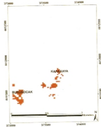
Şekil 16. Çalışılan alanda Aster uydü verisinde Adaptive Sınıflaması ile elde edilen görüntü.
