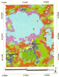
Şekil 18. Çalışılan alanda Aster uydu verisinde K Means Sınıflaması ile elde edilen görüntü .
