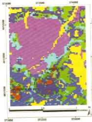
Şekil 16. Çalışılan alanda Aster uydü verisinde Adaptive Sınıflaması ile elde edilen görüntü.
