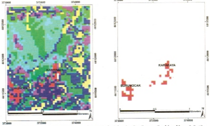
Şekil 9. Çubuklan alanda Landsat uydu verisinde Adaptive Sınıflaması ile elde edilen görüntü.
