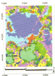
Şekil 12. Çalğalan alanında Aster uydu verisinde Isodata Sınıflaması ile elde edilen görüntü.
