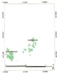
Şekil 5. Çalışılan alanda Landsat uydu verisinde Isodata Sınıflaması ile elde edilen görüntü.
