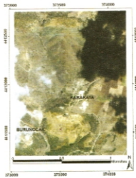
Şekil 20. Çalışılan alanın İkonos RGB123 görüntüsü-kompoziti.
