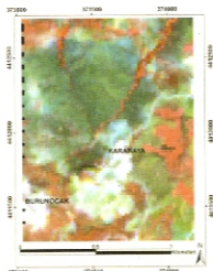
Şekil 11. Çalğalan alanının Aster RGB 321 görüntüsü.
