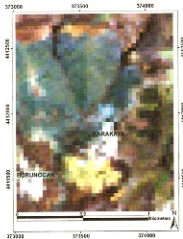
Şekil 2. Çalışılan alanın Landsat RGB 531 kompoziti.
