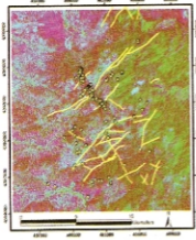
Şekil 14. Çalışma alanındaki tektonik hatların ve numune yerlerinin, Crosta tekniğinin, Landsat 7 ETM+ uyduru verisi dört band için uygulanması ile elde edilen R(PC4),G(PC4 ve PC2'den oluşturulan PC),B(PC2) kompoziti ile elde edilen görüntü üzerindeki konumu.
