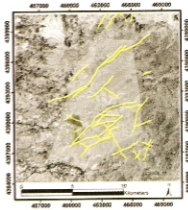
Şekil 16. Çalışma alanındaki tektonik hatların ve numune yerlerinin, Crosta tekniğinin Landsat 7 ETM+ uyduru verisi, dört band için (1,4,5 ve 7) uygulanması ile elde edilen hidroksil (PC4) görüntüsü üzerinde, numunelerden elde edilen Çinko değerleri ile oluşturulan TIN görüntüsünün konumu.
