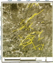
Şekil 4. Çalışma alanının Landsat 7 ETM+ uydu verisi altı bant için PC4 (Hidroksil) görüntüsü ile bölgeden alınan jeokimyasal numunelerin yerleri ve tektonik hatların birlikte sunumu
